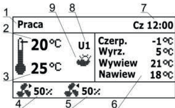
Ekran informacyjny.
